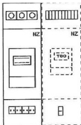
Erweiterung: Anbaukasten mit Klemmstein und Kundenhauptsicherung
