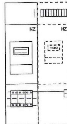
Erweiterung: Sammelschienensystem mit SH-Schalter
