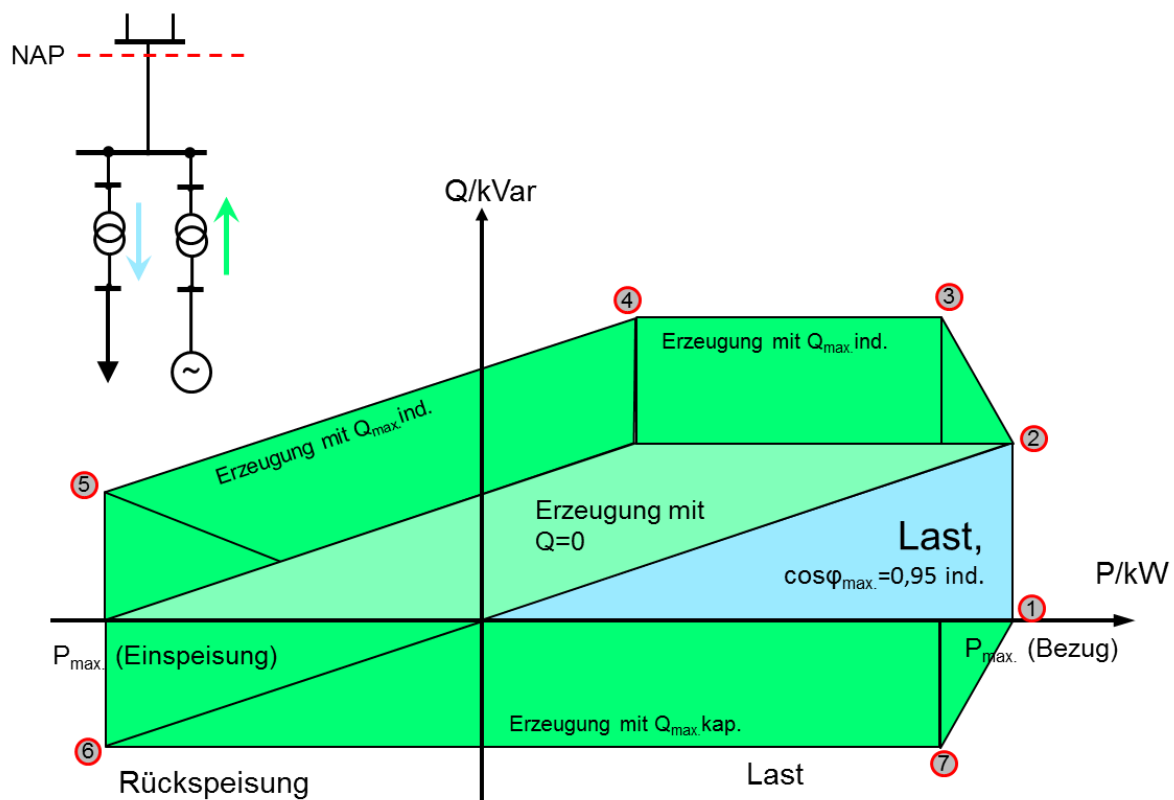
Bild 5.1: Physikalischer Lastfluss am Netzananschlusspunkt beispielhaft für eine Misanlage mit P_{AV,E} \approx 70\% P_{AV,B}
