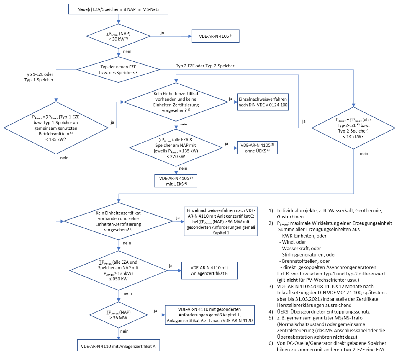
Bild 1.1: Einordnung von Erzeugungsanlagen und/oder Speichern mit Netzanschlusspunkt im Mittelspannungsnetz: Welche VDE-Richtlinie mit welchen Anforderungen ist anzuwenden?
