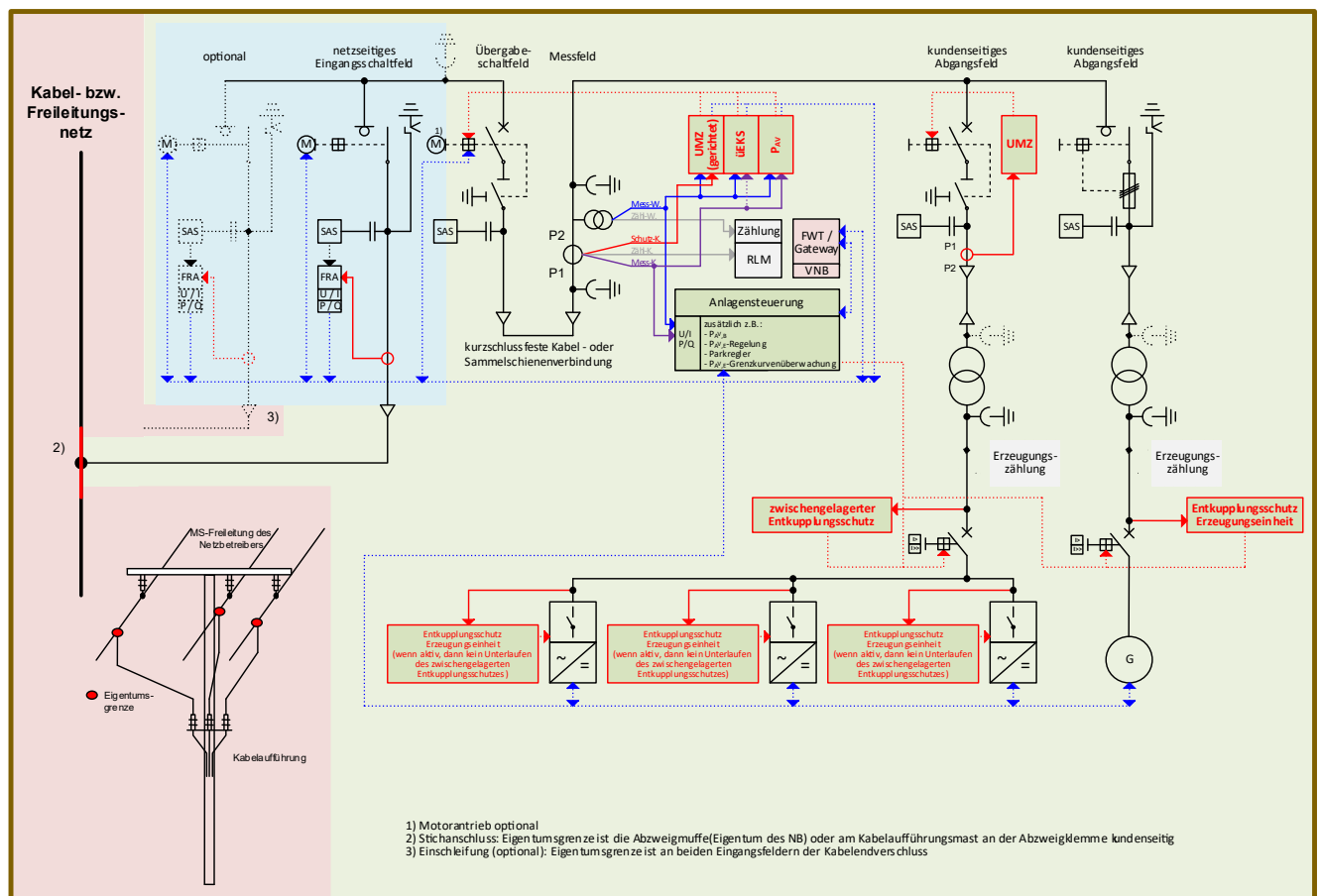
Bild D.4 Ergänzung zu Bild D3 (K)K-LM-LT des BDEW-Musterwortlauts [7]: MS-Erzeugungsanlage – Übergabeschalter als Leistungsschalter, mehrere kundenseitige Transformatorenfelder und zwichengelagerter Entkuppungsschutz
